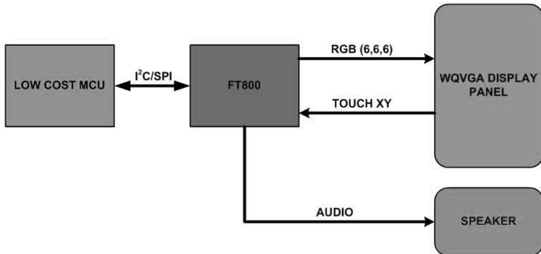
图 2-2FT800 系统设计框图
