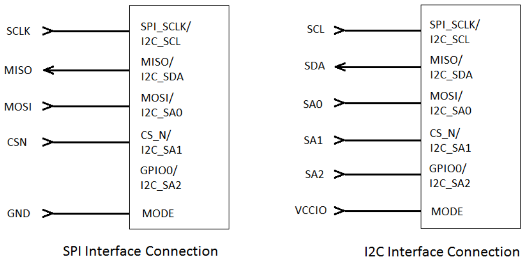
图 4-1 主机接口选项的连接方式
