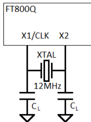
图 4-4 晶体振荡器的连接方式
