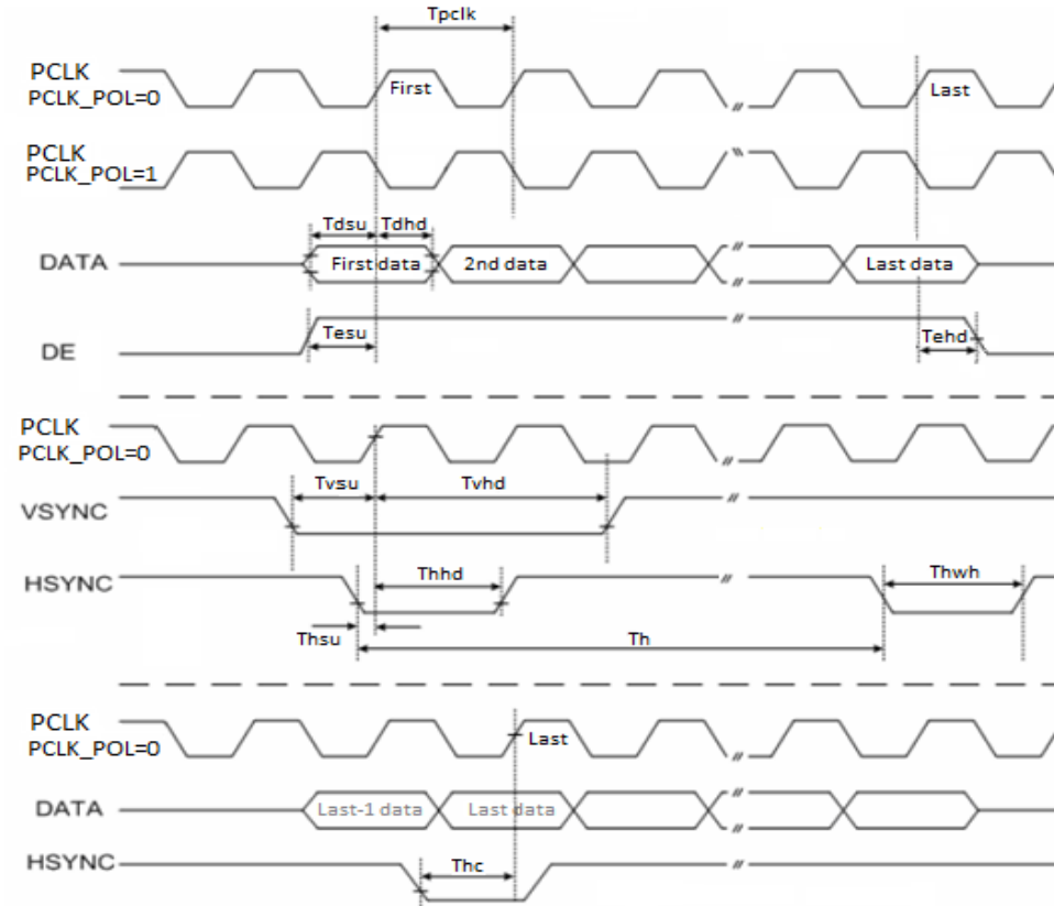
图 6-2 RGB 图像信号时序
