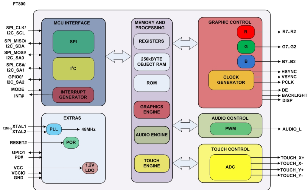
图 2-1FT800 方框图
