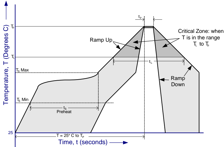
图 8-2 FT800 回流焊温度曲线
